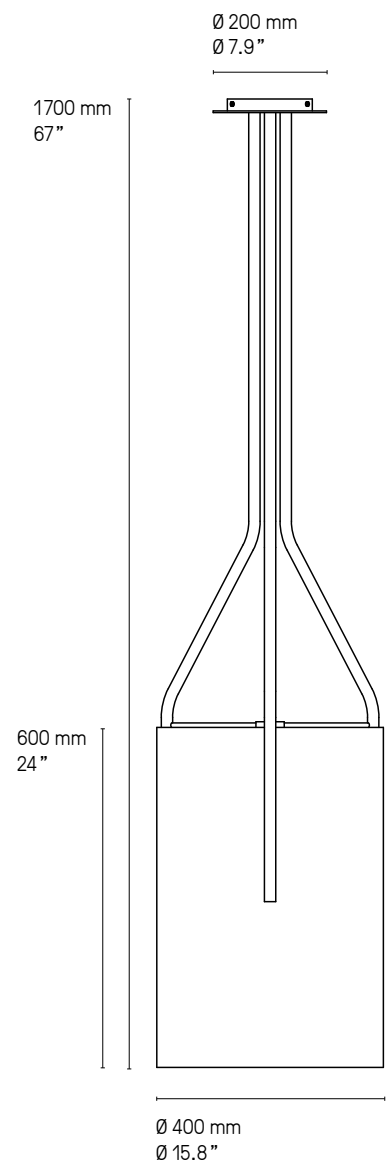
Suspension – Pendant XL
