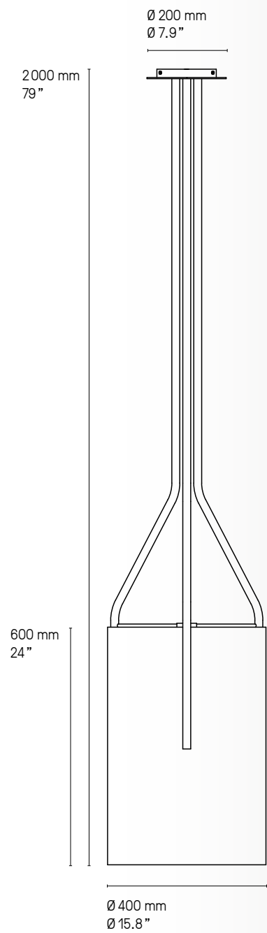
Suspension – Pendant XXL
