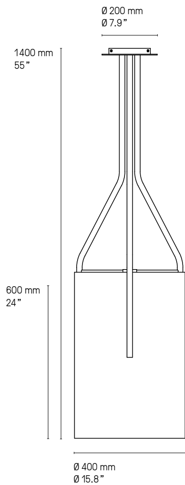
Suspension – Pendant L
