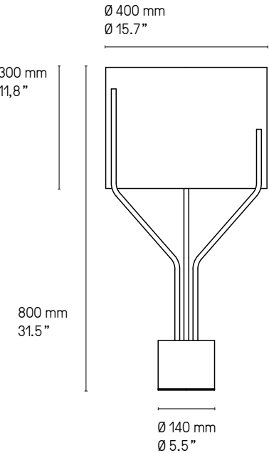
Lampe de table – Table lamp XL
