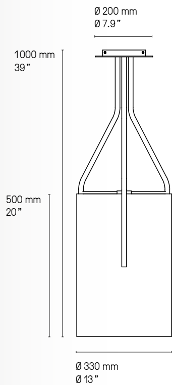
Suspension – Pendant XXS
